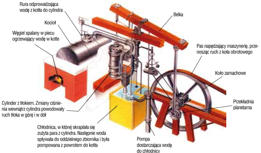
4. Silnik parowy Jamesa Watta (czytaj: dżejmsa łoża) zaprojektowany w 1777 r. stał się główną maszyną napędową. Na podstawie rysunku opisz zasadę działania maszyny parowej
