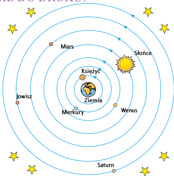
system geocentryczny
