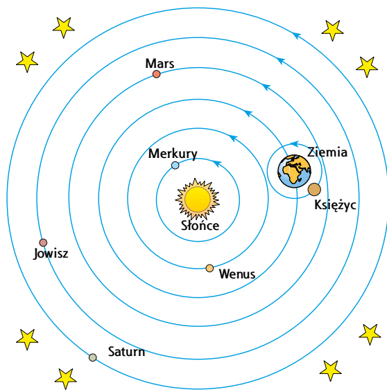
system heliocentryczny
